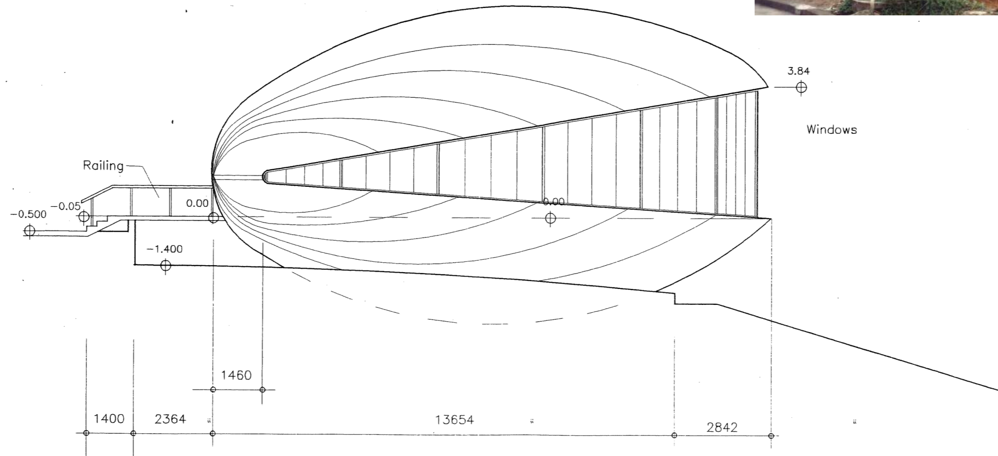
ELEVATION B 1:100
